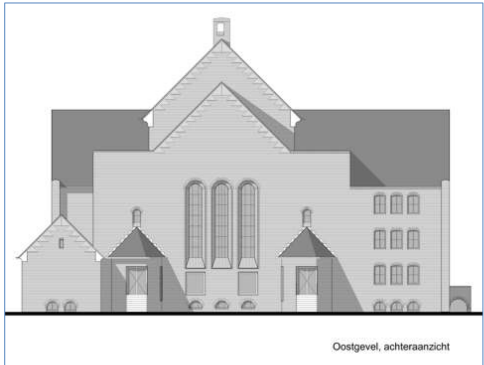
Figuur 6. Gevelaanzichten
