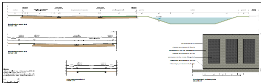
Figuur 12 Doorsnede wadi
