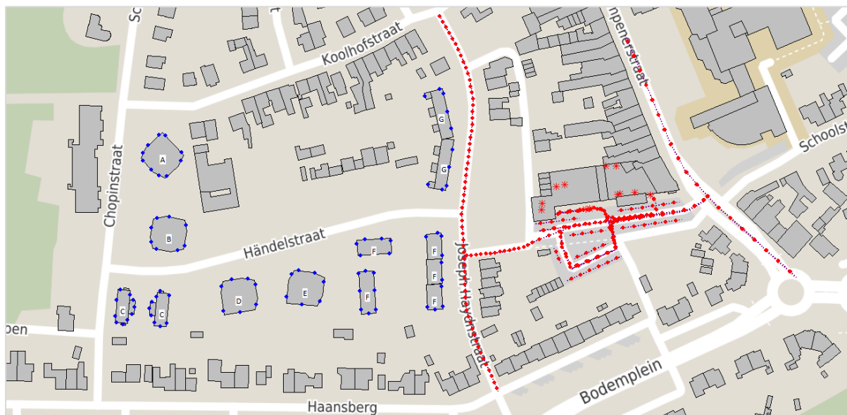
Figuur 3.1 Situering toetspunten en geluidsbronnen.
